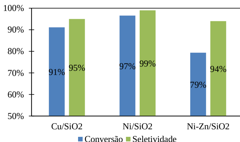
Figura 6 - Valores de Conversão e Seletividade para os melhores catalisadores preparados.
