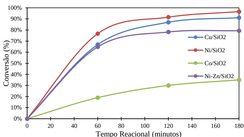
Figura 5 - Perfil reacional para os catalisadores estudados. Pressão: 80 bar; Temperatura: 230°C.
