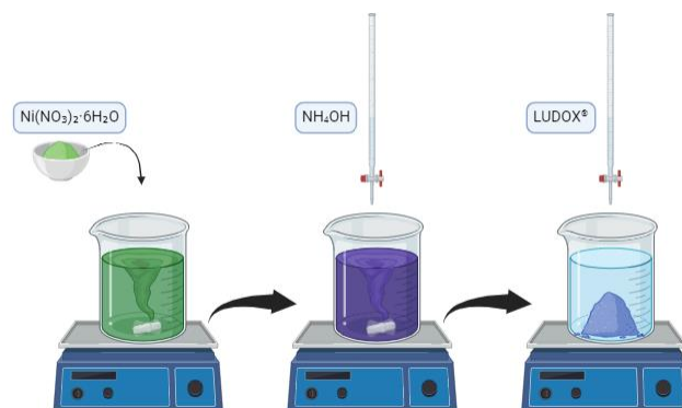
Figura 2 - Procedimento de síntese dos catalisadores estudados. Fonte: O autor (2024).
