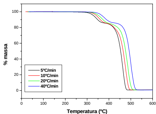
Figura 4. Curvas termogravimétricas do EVA em N 2
