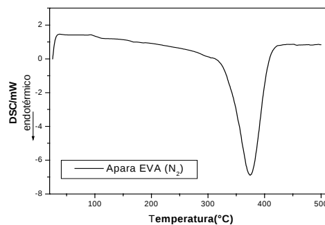
Figura 2. Curva de DSC do EVA em apara em N 2
