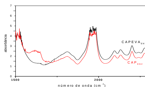
Figura 10. Espectros FTIR do CAPEVA e do CAP envelhecidos
