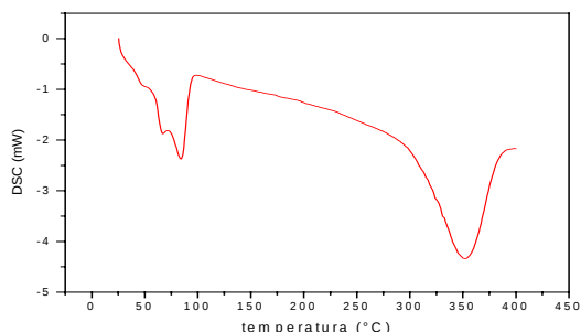
Figura 1. Curva de DSC do EVA em N 2
