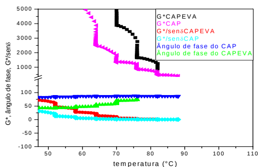
Figura 11. Ensaios dinâmicos mecânicos do CAPEVA e CAP
