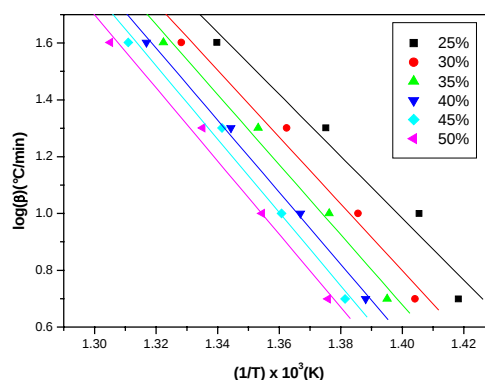
Figura 7. Gráfico do EVA em N 2
