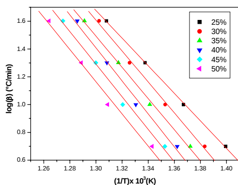
Figura 6. Gráfico do EVA aparas em N 2
