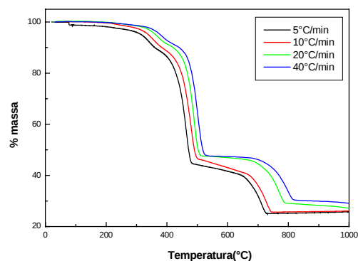
Figura 5. Curvas termogravimétricas do EVA aparas em N 2
