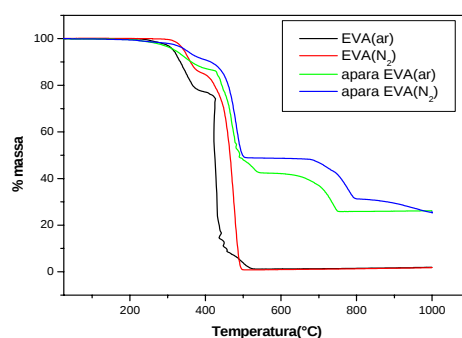
Figura 3. Curvas termogravimétricas do EVA e de EVA aparas em atmosfera de ar e N 2
