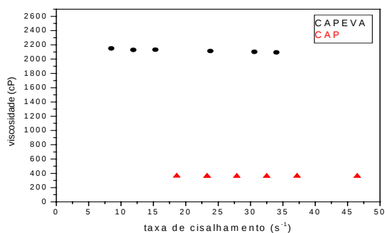
Figura 8. Viscosidade do CAPEVA e CAP
