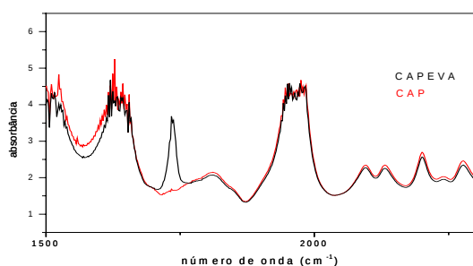
Figura 9. Espectros FTIR do CAPEVA e CAP
