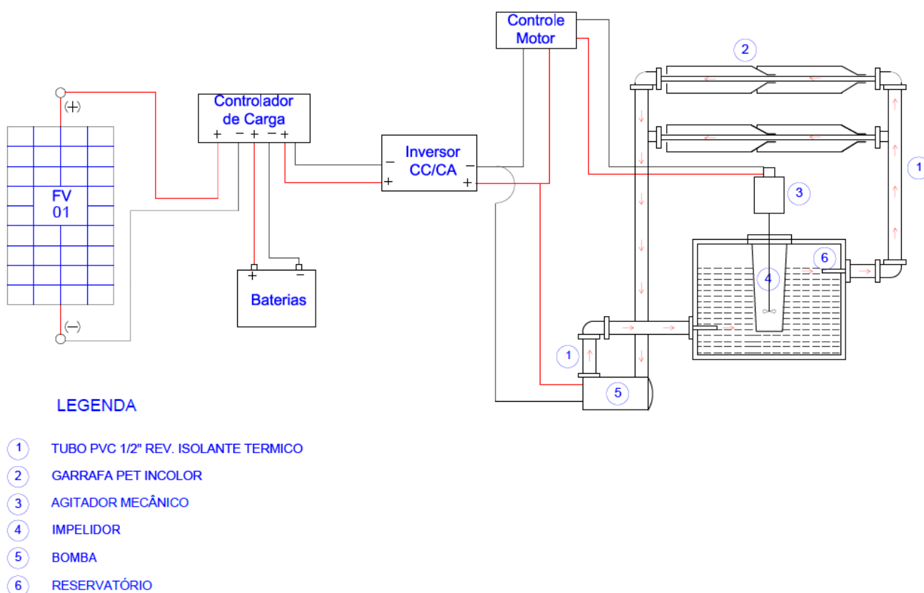
Figura 4 – Esquema do sistema conforme aplicação real. Fonte: Autoria própria.
