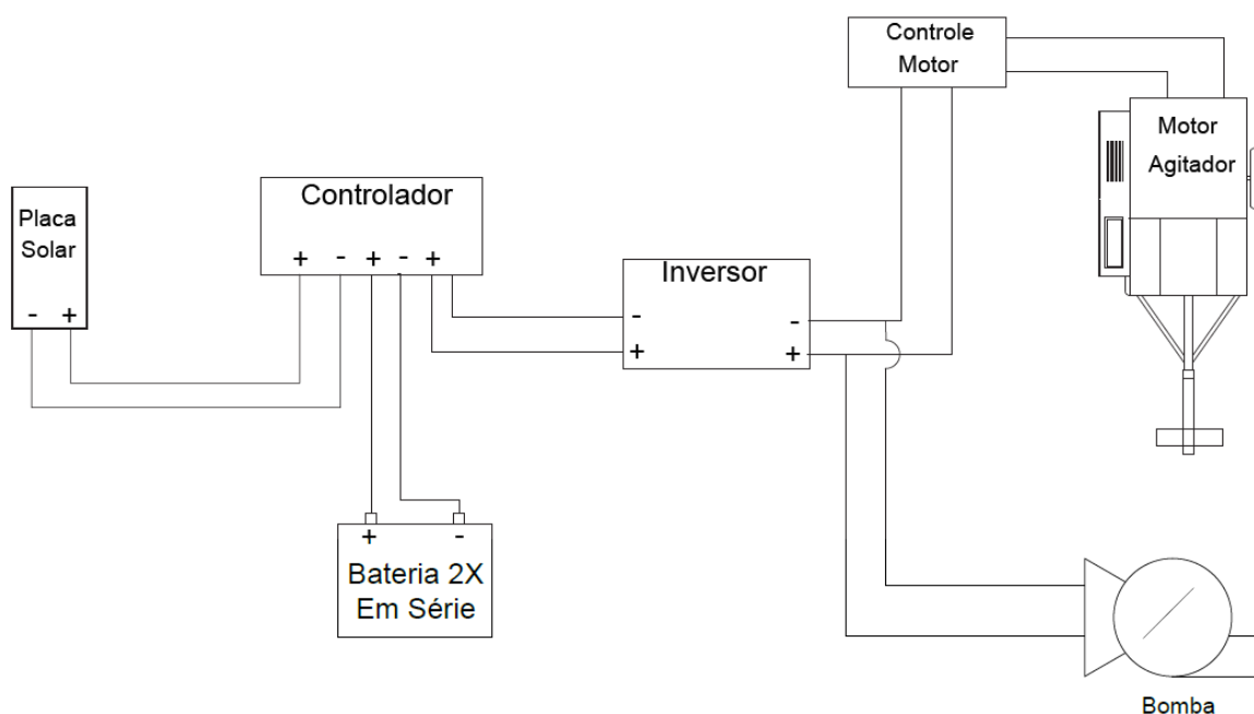
Figura 1 – Esquemática do circuito elétrico utilizado no protótipo. Fonte: Autoria própria.
