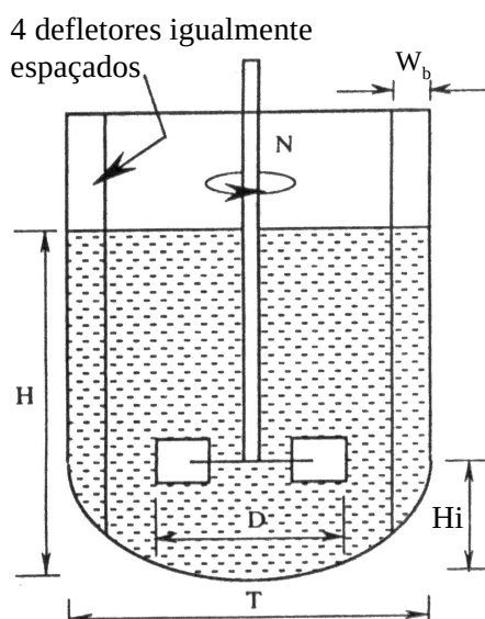
Figura 2 – Dimensões do reator construído. Fonte: Autoria própria.
