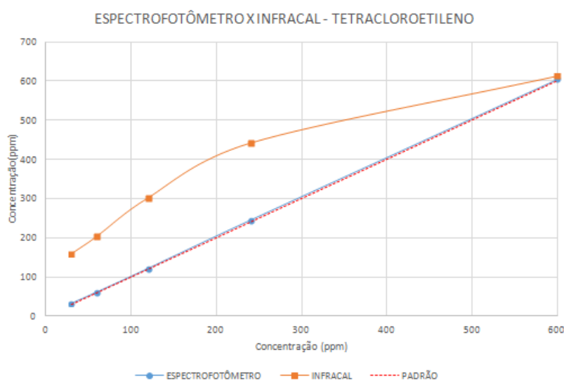
Figura 3: Espectrofotômetro x Infravermelho - Tetracloretileno.
