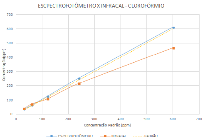
Figura 4: Espectrofotômetro x Infralcal-Clorofórmio
