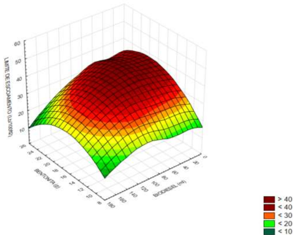
FIGURA 4. Influencia da quantidade de bentonita e biodiesel no limite de escoamento do fluido de perfuração.
